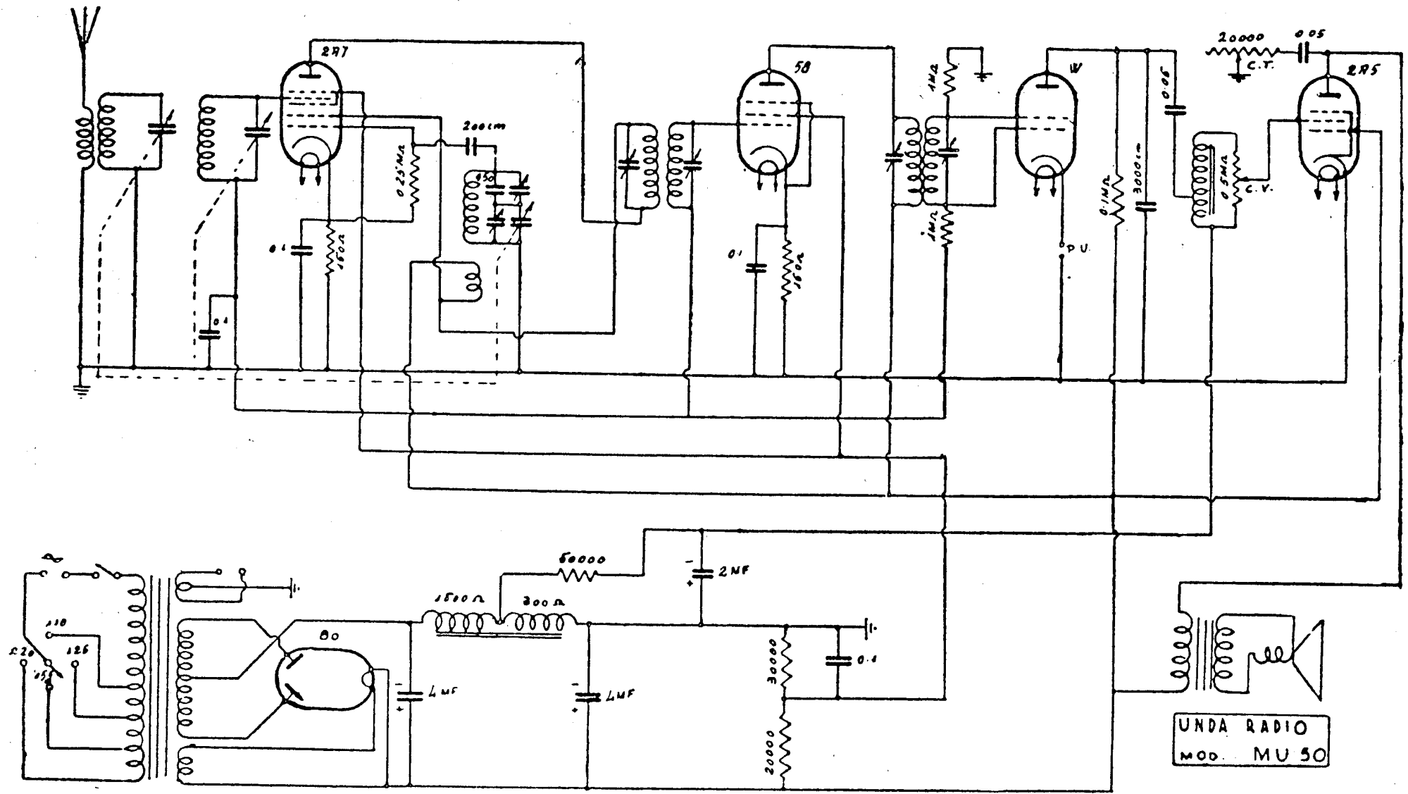
UNDA RADIO. — Modello « M. U. 50 ». - Produzione 1933. - Media frequenza: 175 kc.
